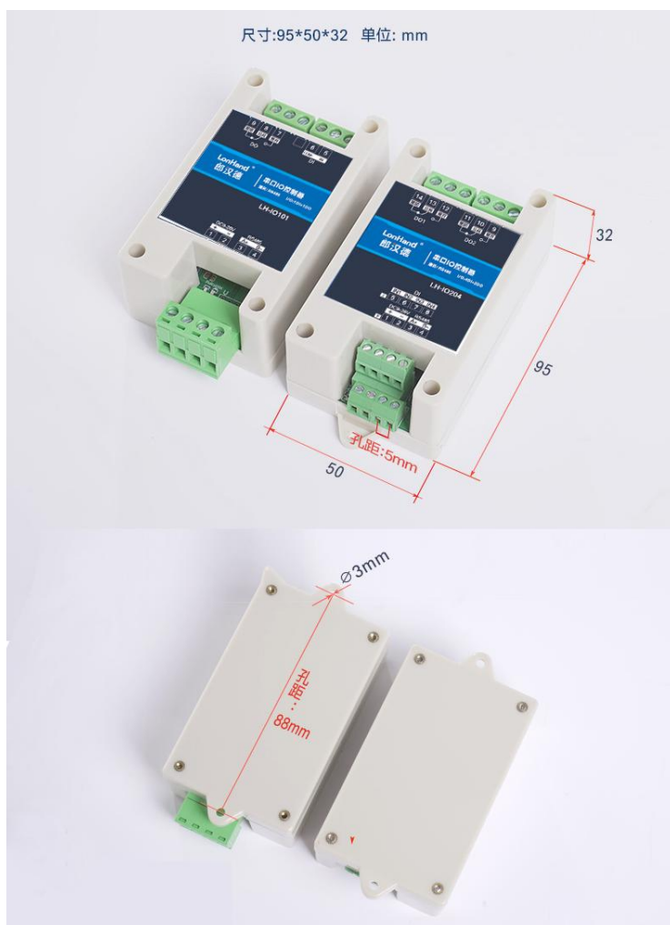
产品尺寸图
